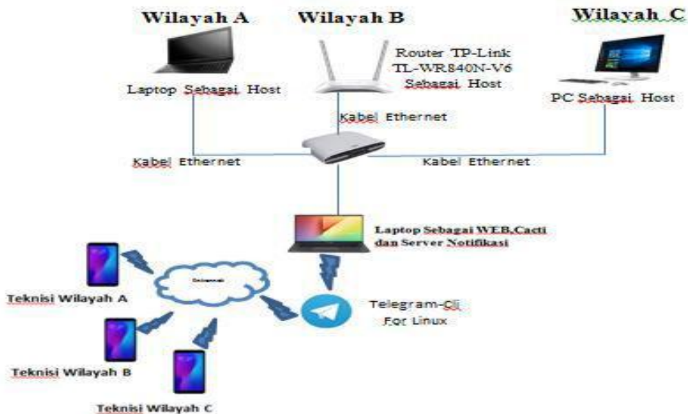
Gambar 6. Arsitektur pengujian
