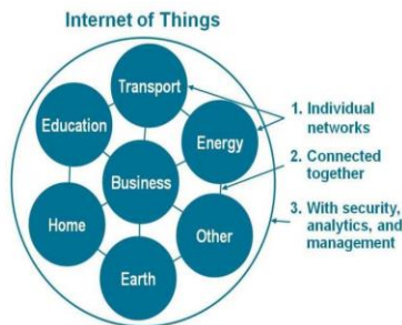
Gambar 4 IOT
