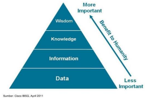
Gambar 3 Piramida pengetahuan
