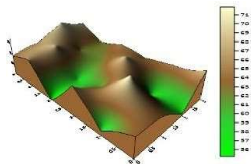
Gambar 3 : Contour Map SPL Ruang Aula 3D Menggunakan Loudspeaker
